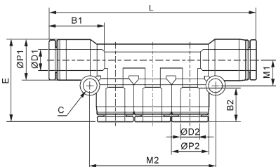
EPKG 減徑五通 Union
